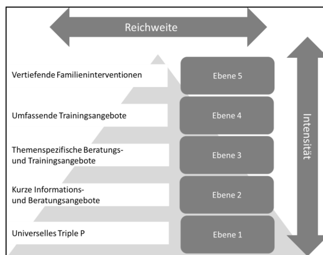
Abbildung 2: Mehrebenen-Modell
